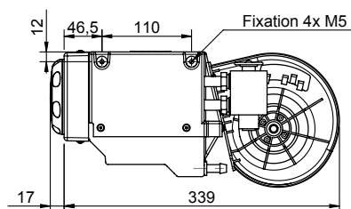
HVAC
